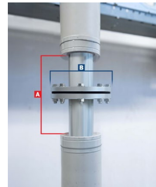
Figuur 4: Flens
